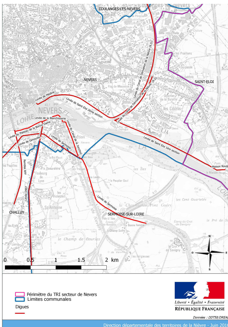
Illustration 8: Ouvrages de protection de l'agglomération de Nevers (noms des ouvrages)
