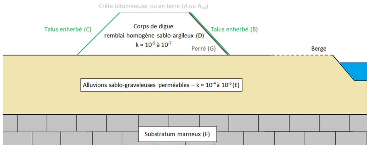
Figure 15 : Profil non renforcé sans assise imperméable (F1)
