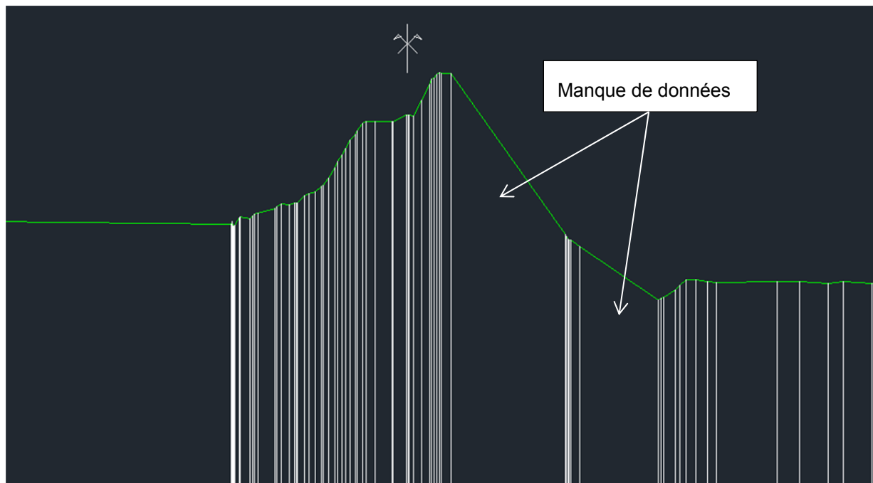
Figure 4: Exemples de profils en travers avec des manques de données importants (profil en travers sur une levée du val de Decize)
