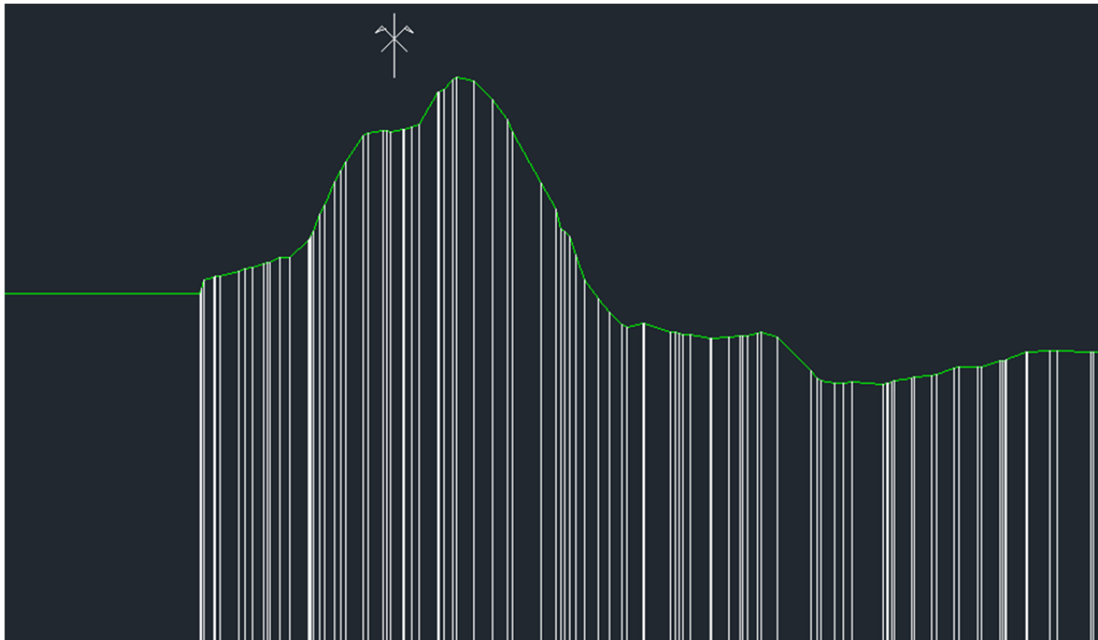
Figure 3 : Exemple de profil en travers type pour le val de Decize (58)
