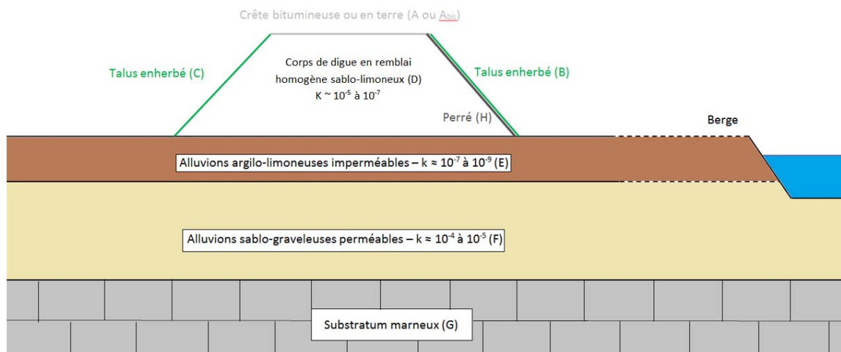
Figure 16 : Profil non renforcé avec assise imperméable (F1)
