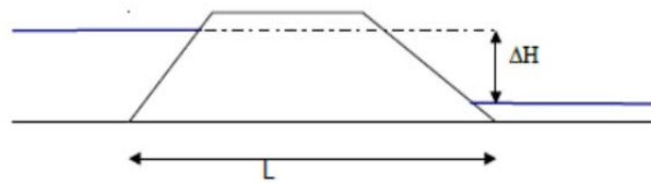
Figure 14 : Schéma de principe pour le calcul du gradient hydraulique de la formule de Bligh
