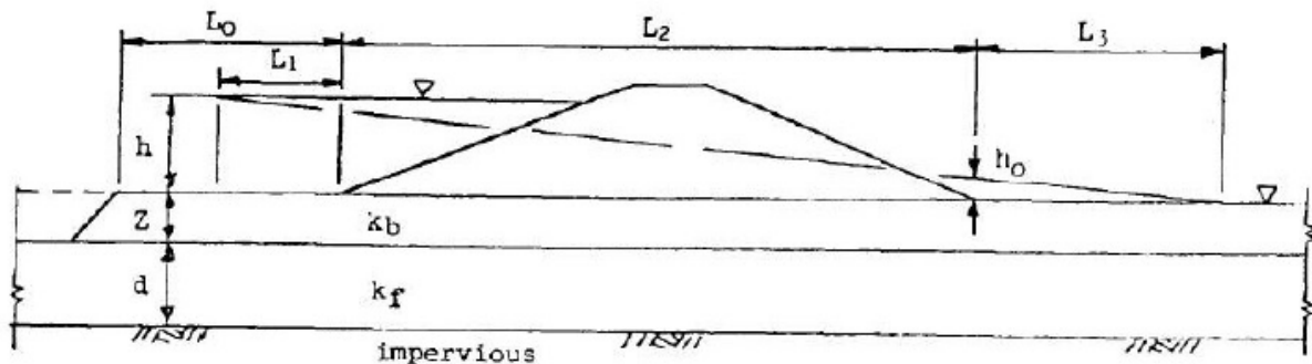
Figure 33 : Schéma type présentant les variables utilisées dans le calcul du coefficient de sécurité F_h du soulèvement hydraulique
