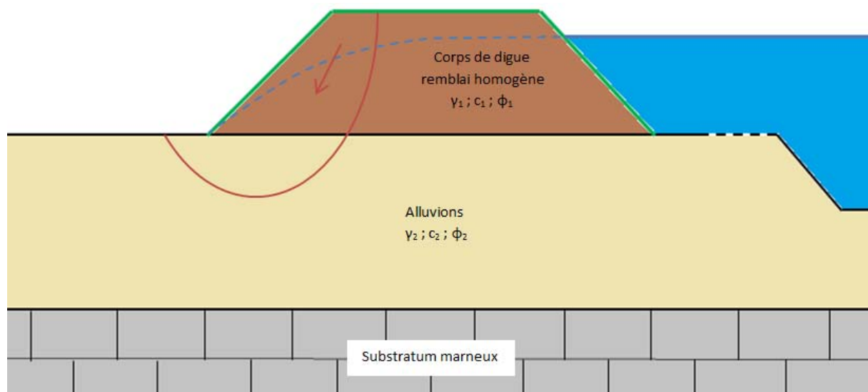
Figure 23 : Schéma de principe d'un glissement de talus sur une digue côté val
